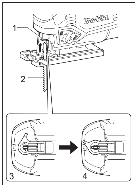
► 1. Porta-útil 2. Hoja de sierra 3. Posición fija 4. Posición liberada
