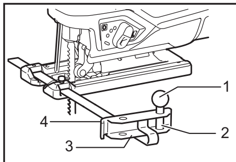
► 1. Perilla roscada 2. Clavija 3. Guía lateral de corte (regla de guía) 4. Guía lateral
