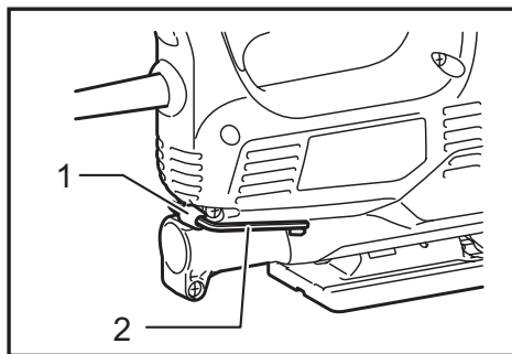
► 1. Portallaves 2. Llave hexagonal
