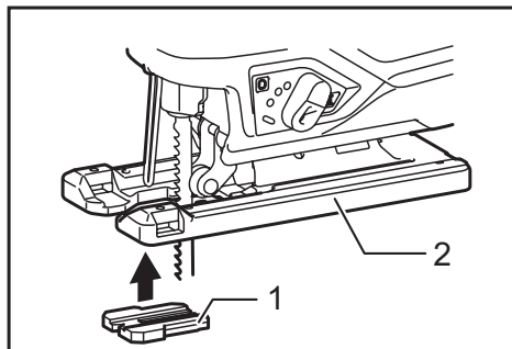
► 1. Dispositivo antiastillado 2. Base de la herramienta
